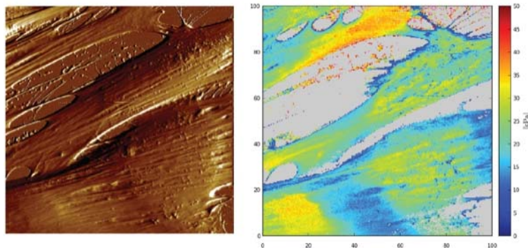
Figure 1: Fibroblastes (cellules du derme) vus en topographie (peak force error, gauche) et en élasticité (module d'Young, droite)
