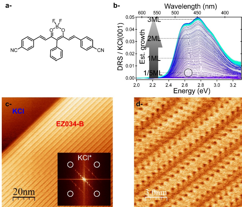
Figure 1 : a-Exemple de tecton moléculaire utilisé pour l'analyse combinée DRS / AFM non-contact. Molécule EZ034-B. b-Spectres DRS de EZ034-B sur KCl(001) de 0 à 3 monocouches (ML). c- Imagerie AFM non-contact de la phase supramoléculaire d'EZ034-B dans le régime 1/5ML sur KCl(001). Les molécules forment des rangées parallèles alignées le long des rangées polaires [110] du substrat. d- Image AFM non-contact haute résolution de la phase supramoléculaire. Sa structure peut conditionnellement permettre l'interprétation de sa réponse optique telle que mesurée en DRS [4].
